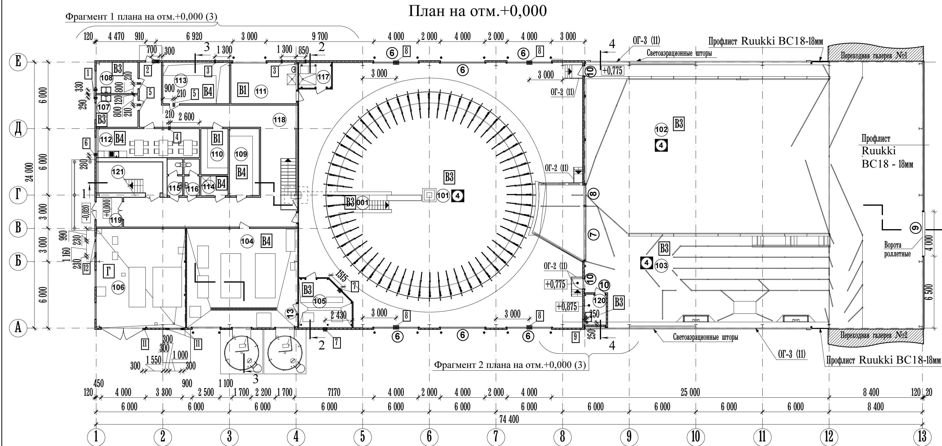
Экспликация помещений план на отм.+0,000
